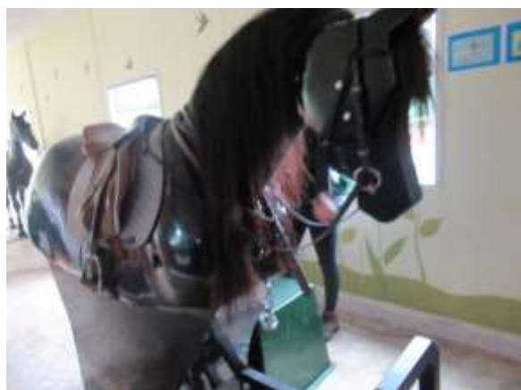
練習用の乗馬ロボット
